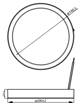
DN027C G3 LED15/NW 15W 220-240V D200
