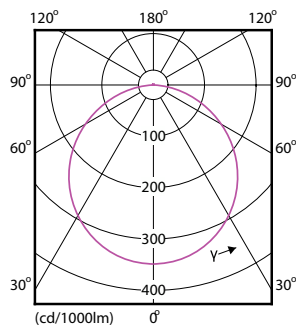
Downlight DN027C G3 LED15 NW 15W D200
